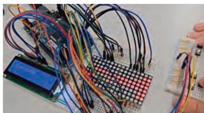
マイコンを使用して作成したゲーム Games created using a microcontroller
