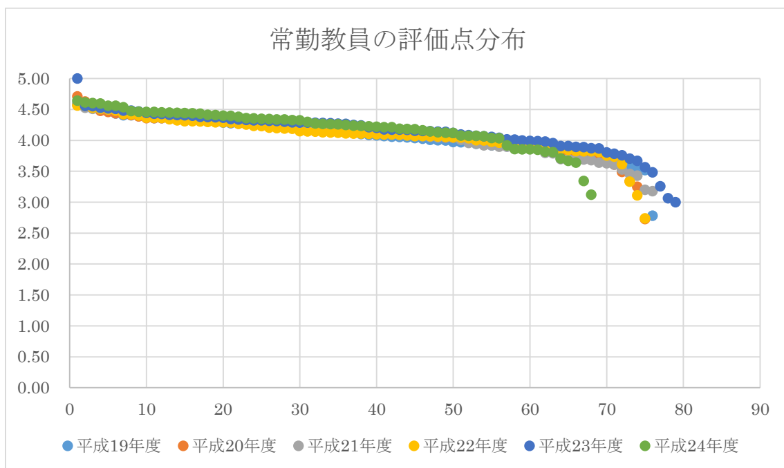
図 1.常勤教員の評価点分布（平成 19 年～平成 24 年）
