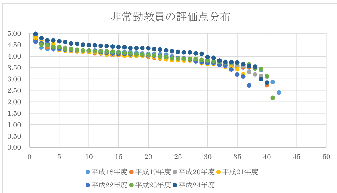
図 2.非常勤教員の評価点分布（平成 18 年～平成 24 年）
