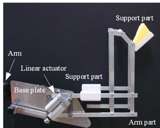
上肢用パワーアシスト装具
