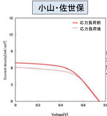
(a)塗布型太陽電池のI-V特性
