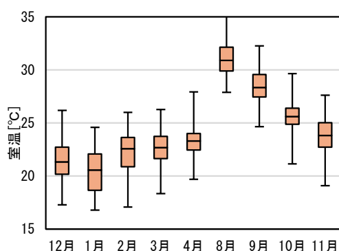
西埜邸室温分布図
