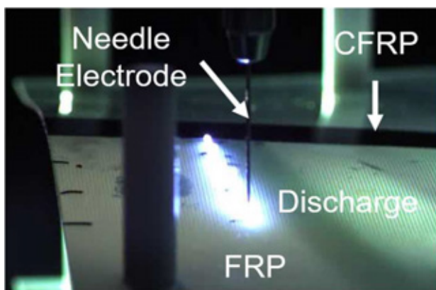
放電試験の様子
