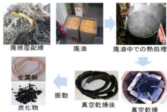
図2 処理プロセスの概略
