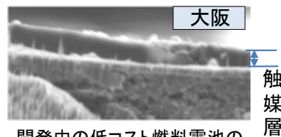
開発中の低コスト燃料電池の触媒層の断面図
